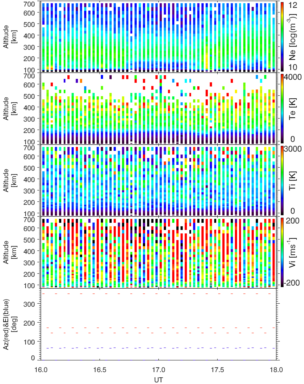
EISCAT 2005-09-02_16_18UT_steffe_ant@32m.
