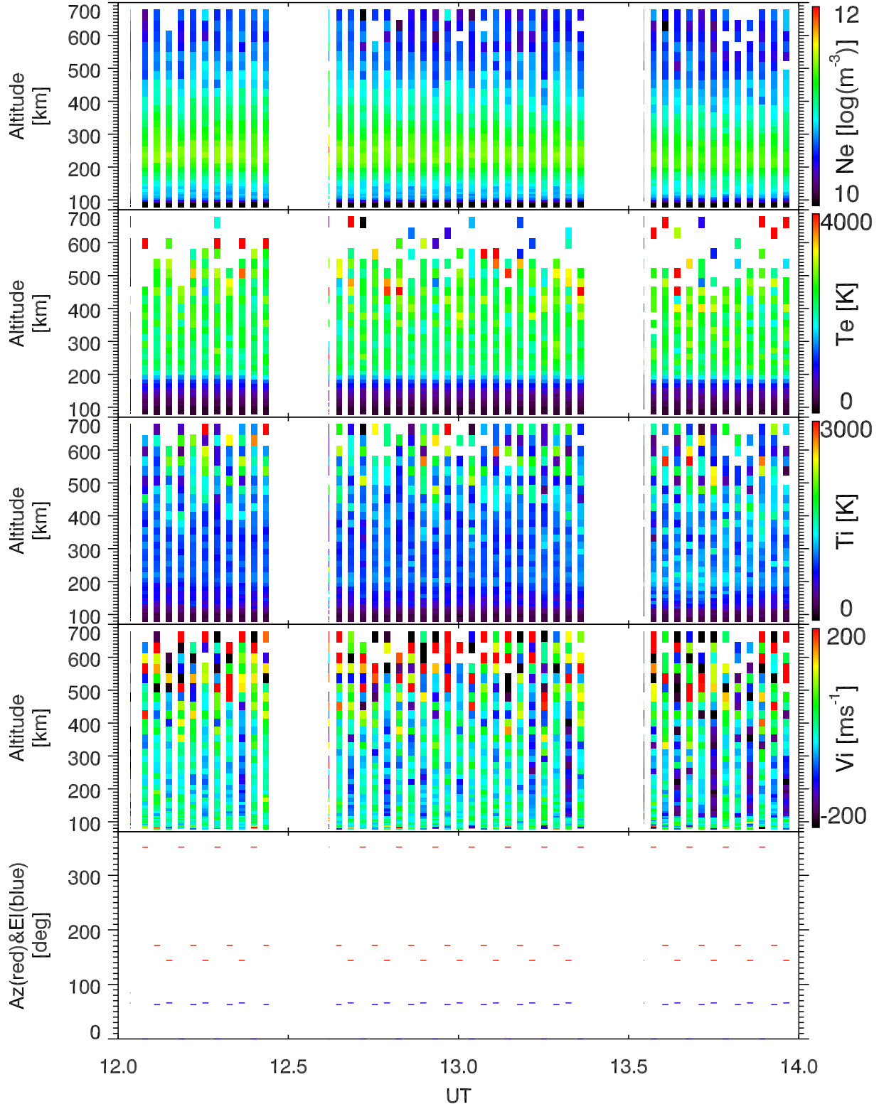
EISCAT 2005-09-08_12_14UT_steffe_ant@32m.
