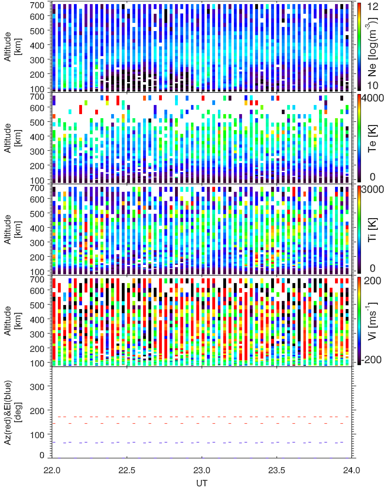
EISCAT 2005-09-15_22_24UT_steffe_ant@32m.
