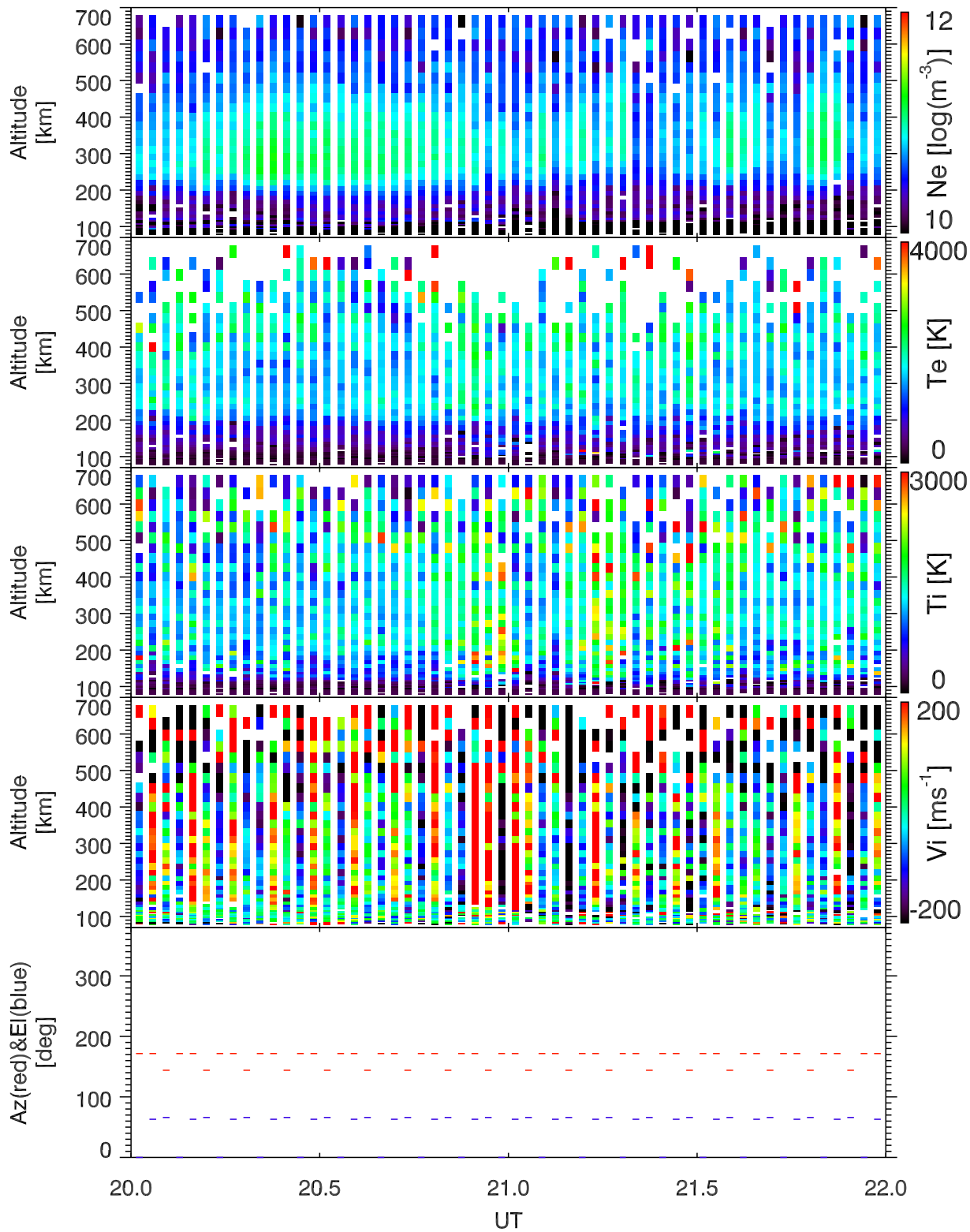
EISCAT 2005-09-19_20_22UT_steffe_ant@32m.
