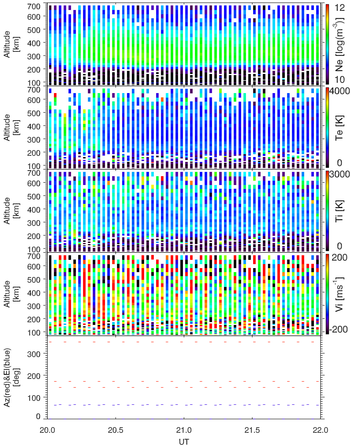
EISCAT 2005-09-25_20_22UT_steffe_ant@32m.
