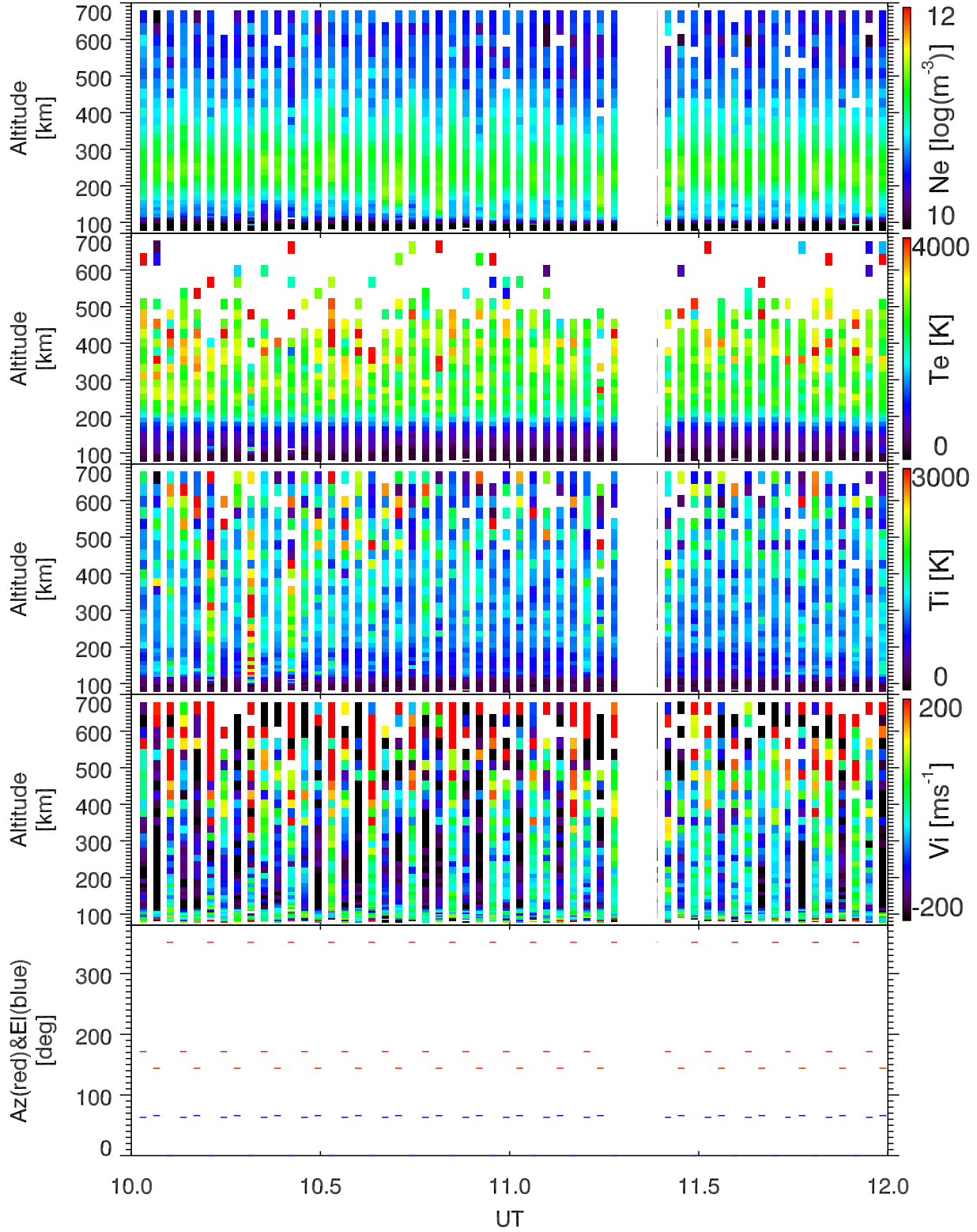
EISCAT 2005-09-27_10_12UT_steffe_ant@32m.
