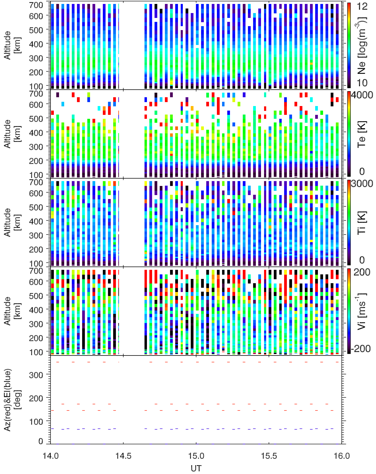
EISCAT 2005-09-29_14_16UT_steffe_ant@32m.
