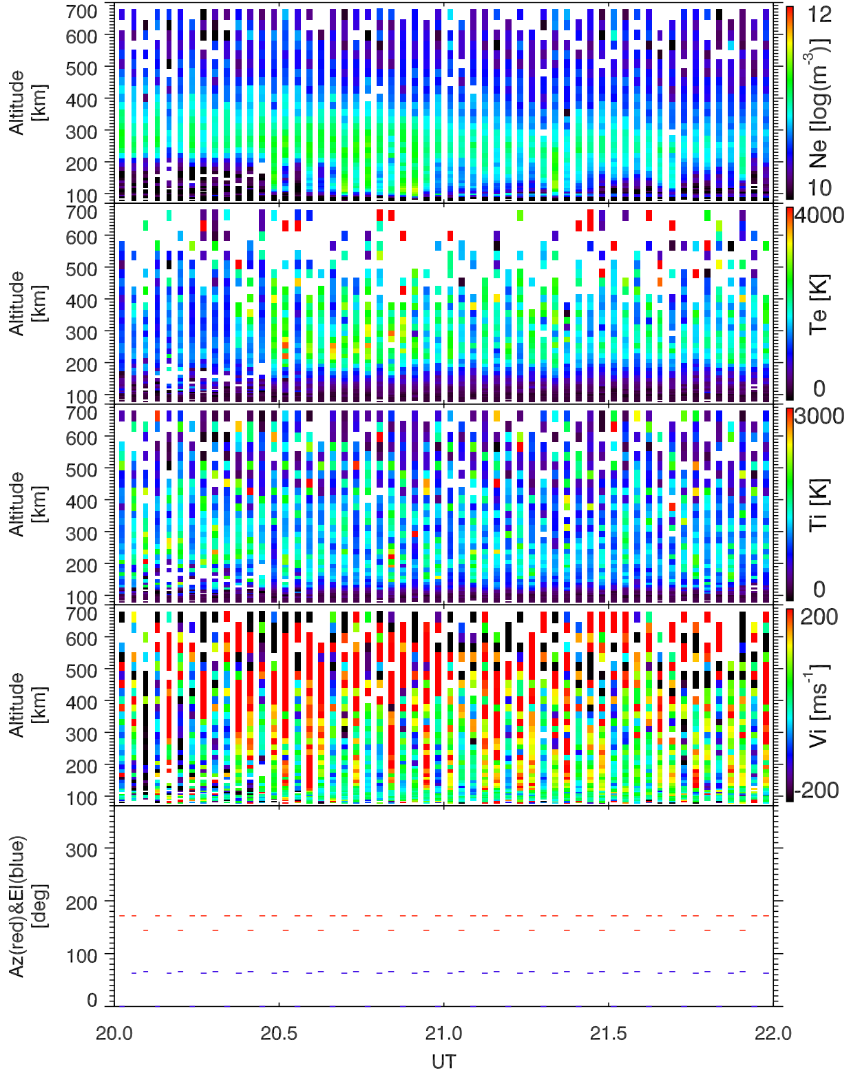
EISCAT 2005-09-29_20_22UT_steffe_ant@32m.
