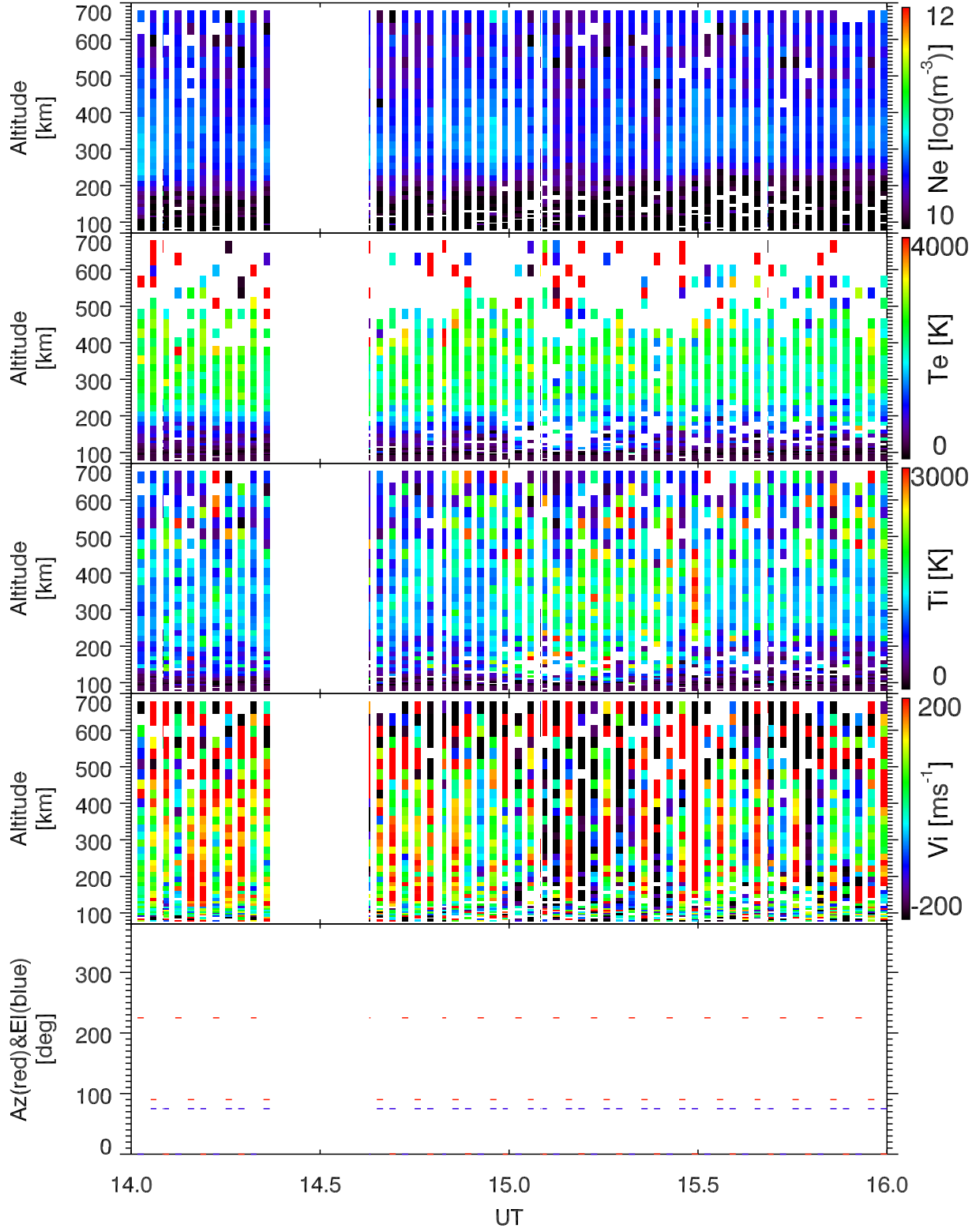
EISCAT 2006-02-21_14_16UT_steffe_ant@32m.
