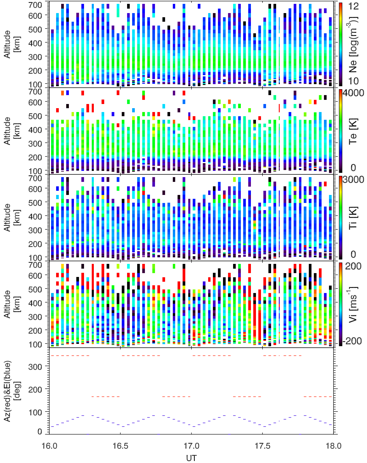
EISCAT 2006-09-20_16_18UT_tau0_ant@32m.
