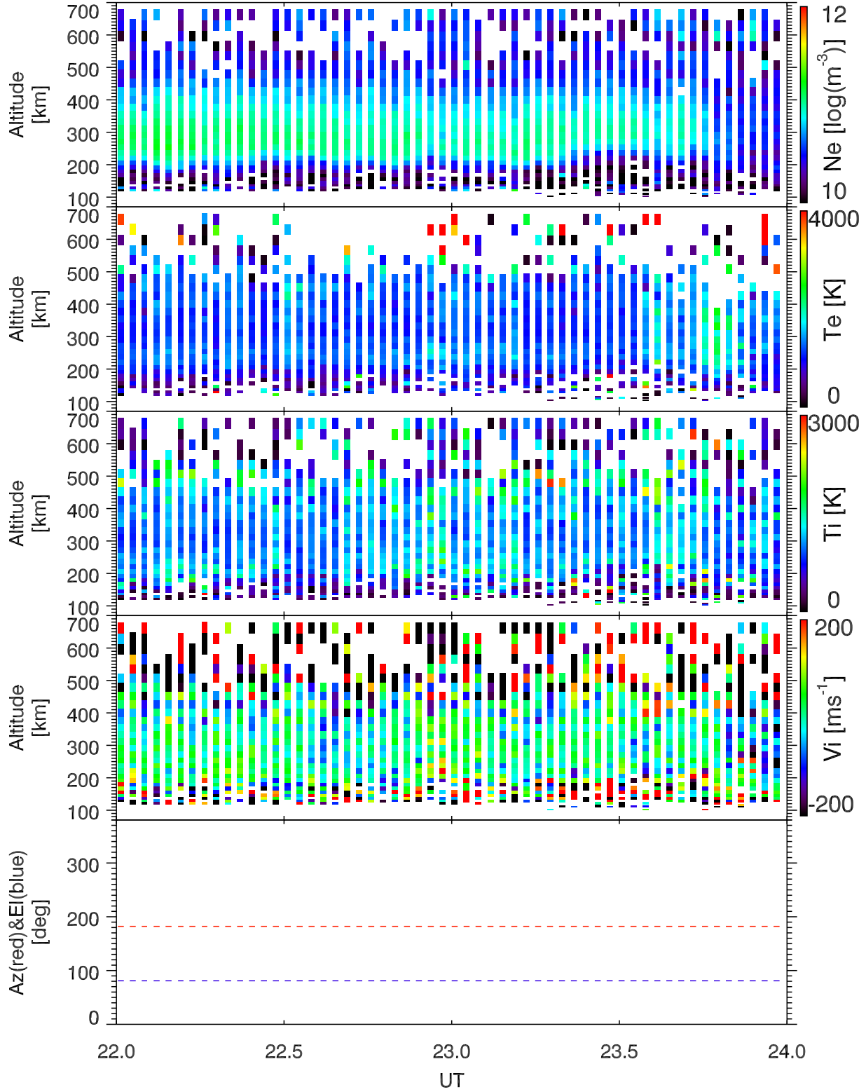
EISCAT 2006-09-20_22_24UT_tau0_ant@42m.
