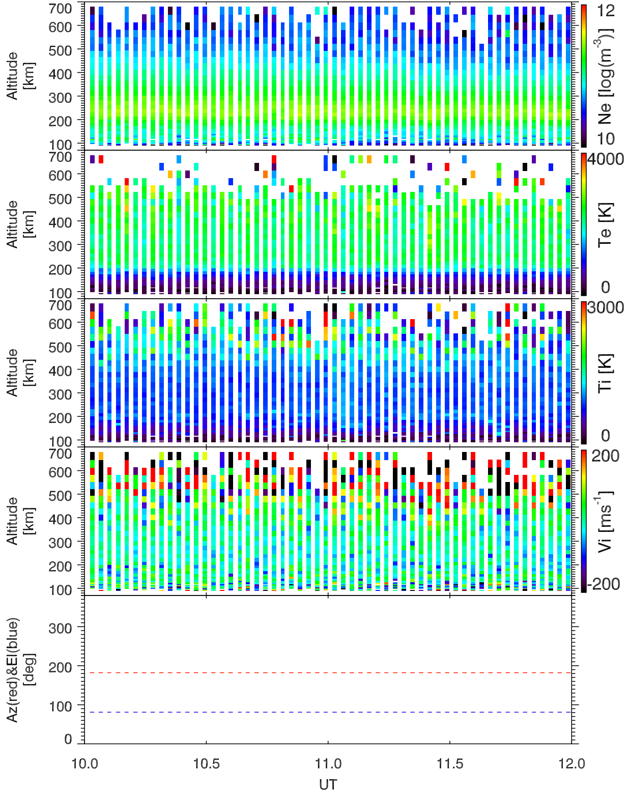
EISCAT 2006-09-21_10_12UT_tau0_ant@42m.
