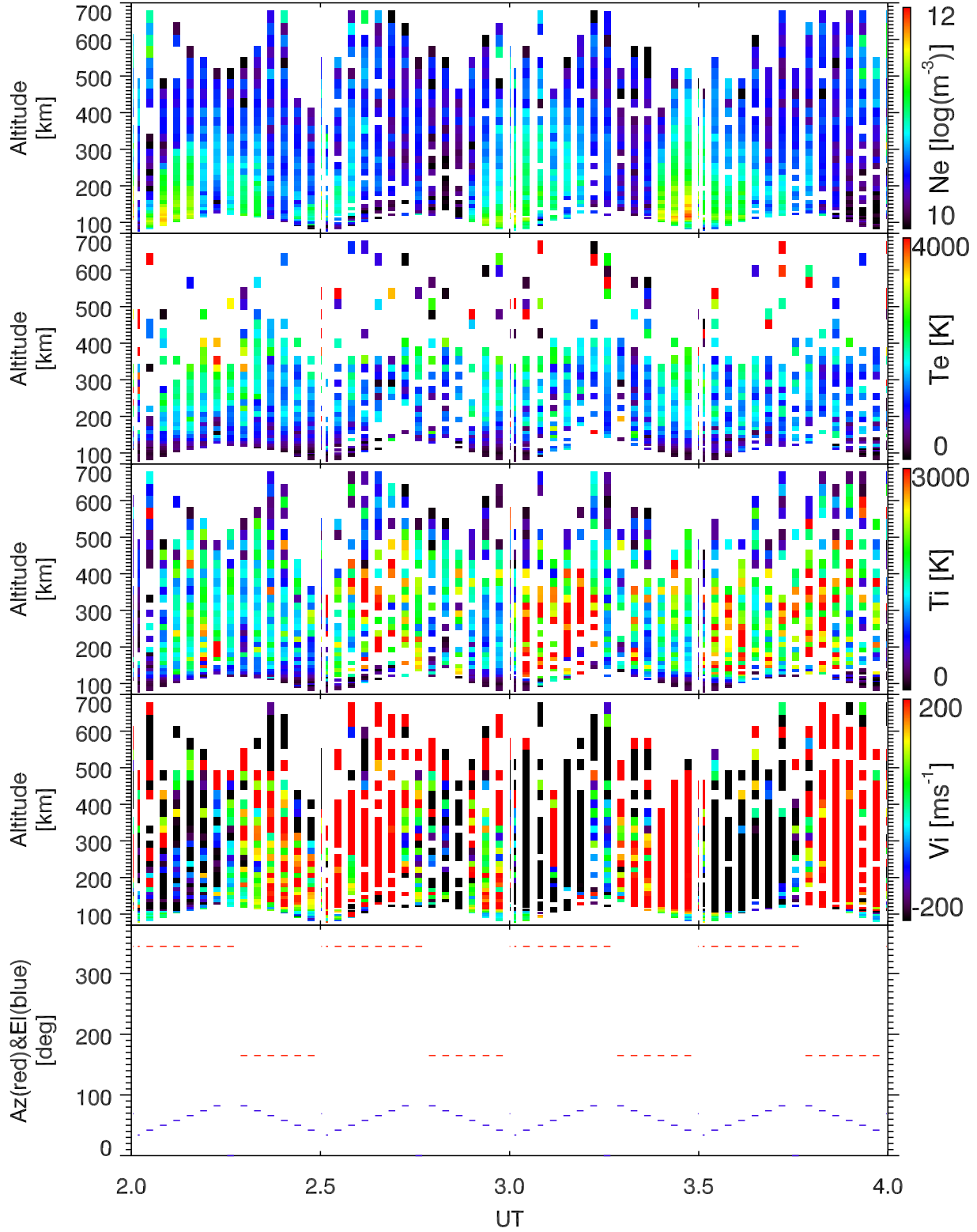
EISCAT 2006-12-15_02_04UT_tau0_ant@32m.
