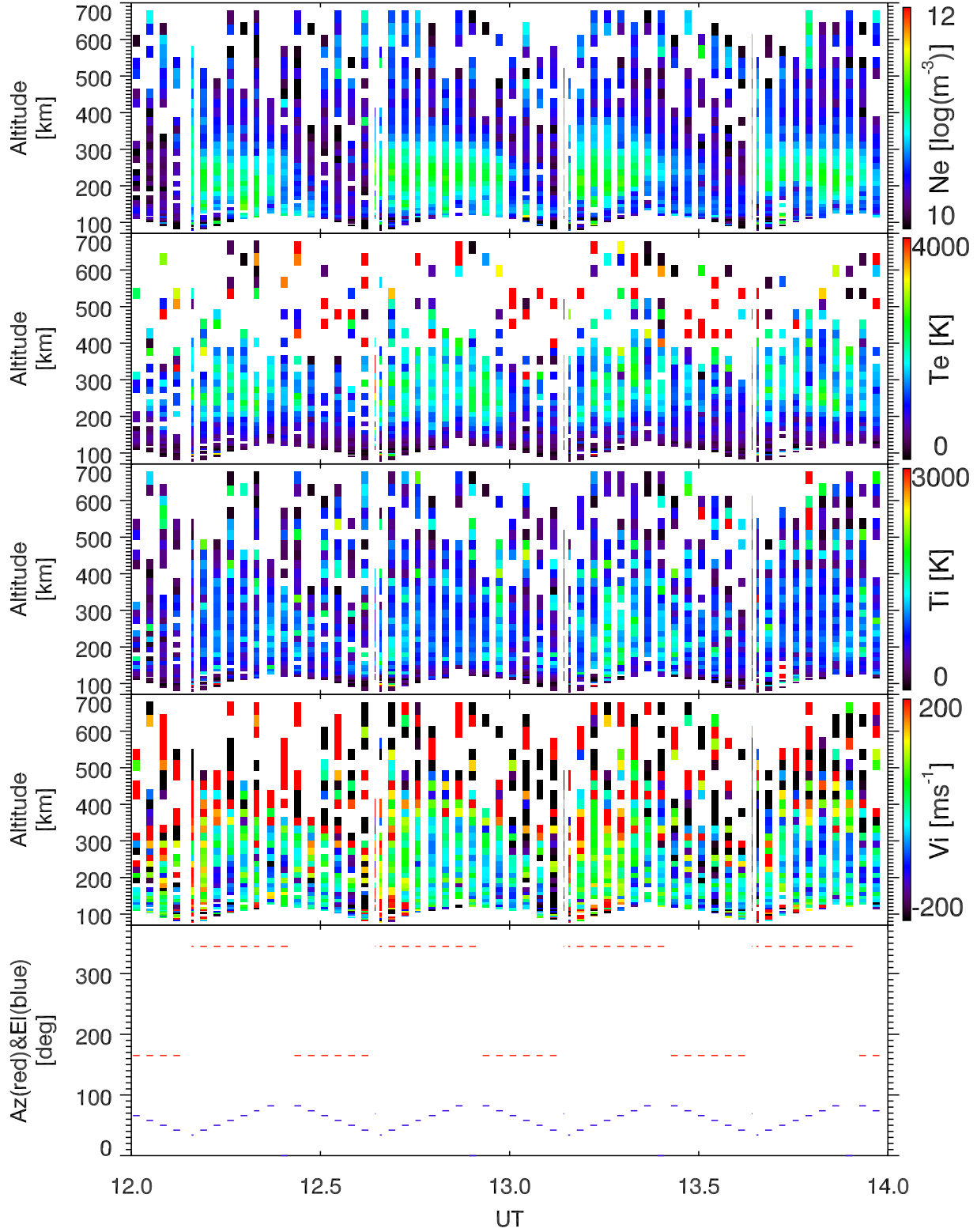
EISCAT 2006-12-16_12_14UT_tau0_ant@32m.
