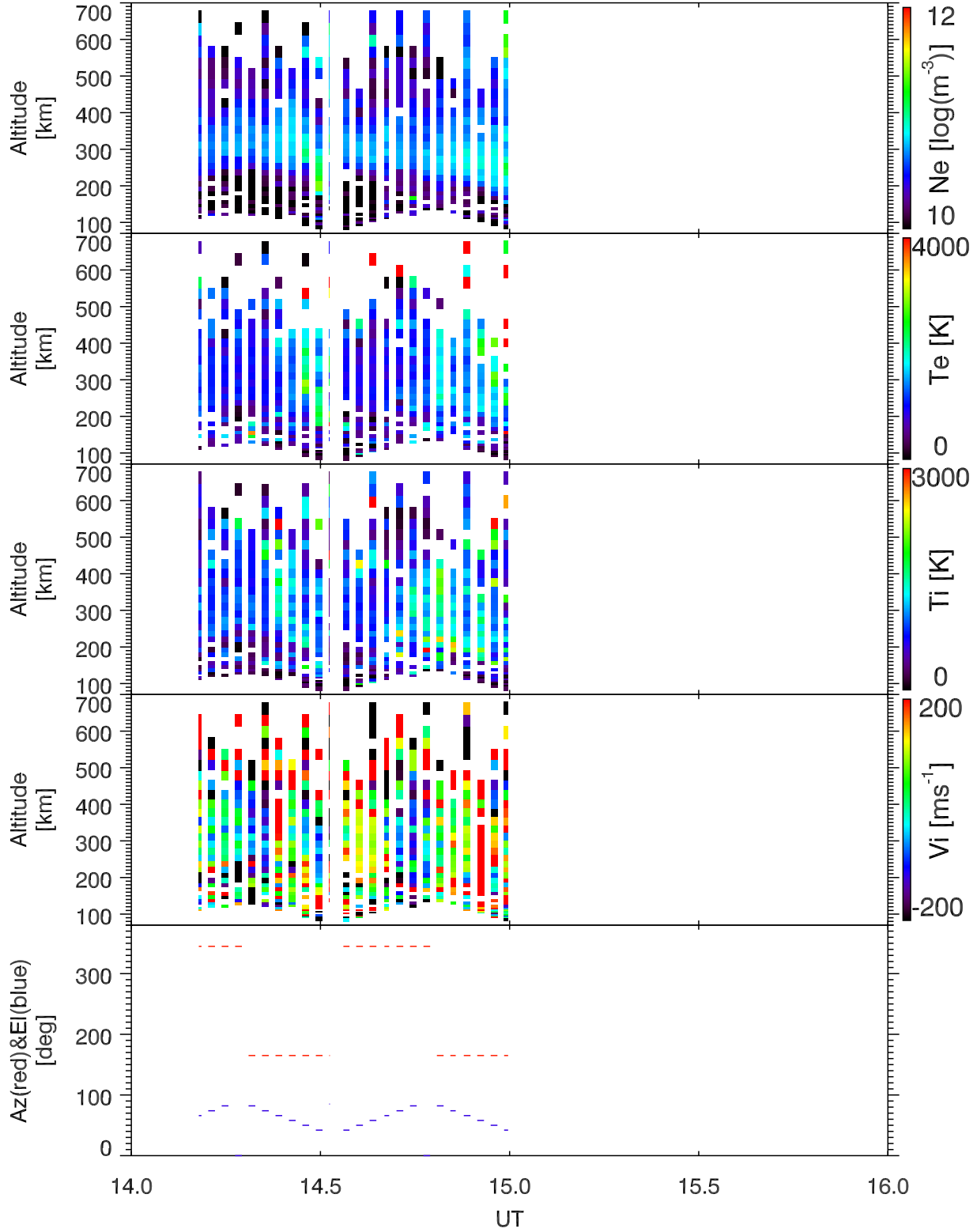
EISCAT 2006-12-19_14_16UT_tau0_ant@32m.
