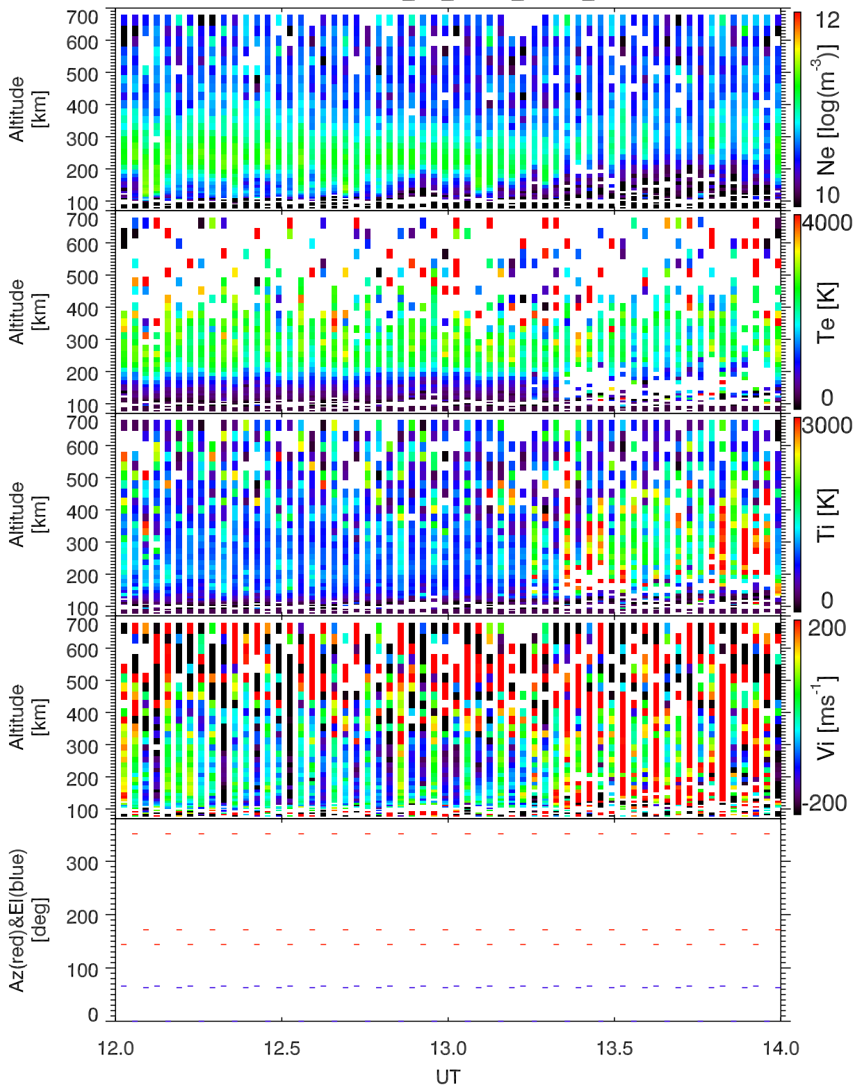
EISCAT 2007-02-07_12_14UT_steffe_ant@32m.
