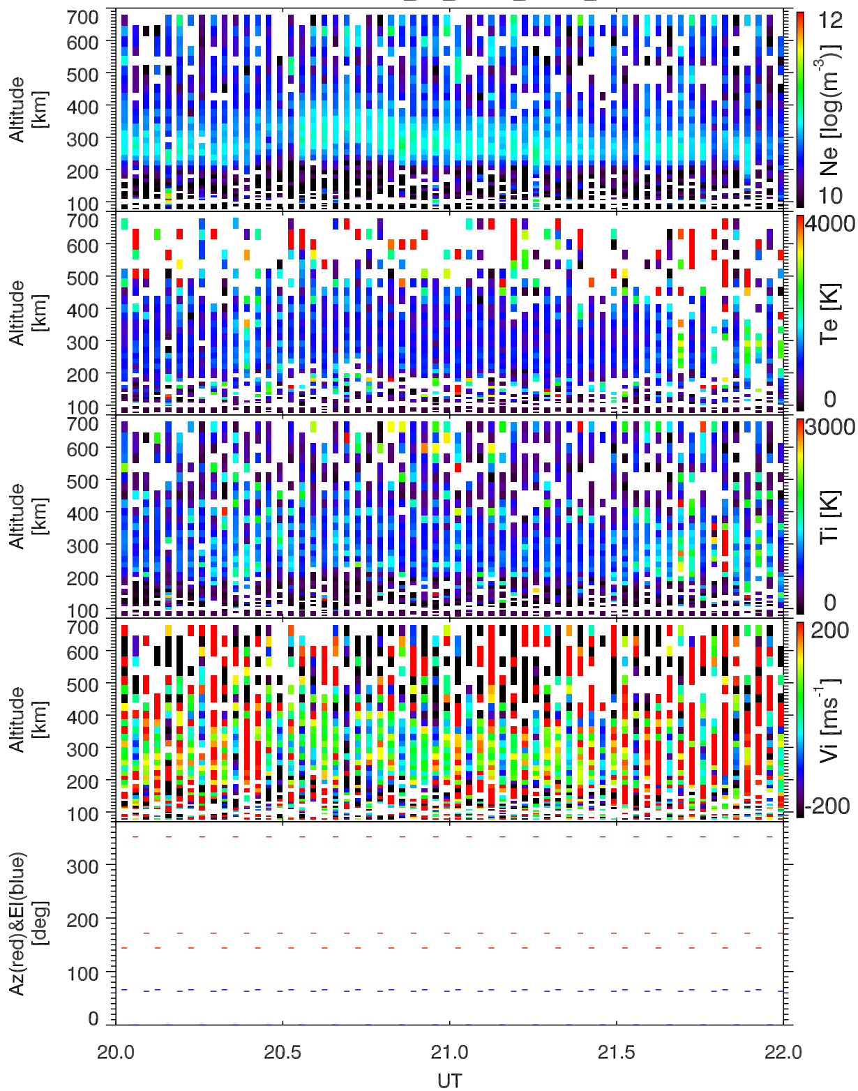
EISCAT 2007-02-08_20_22UT_steffe_ant@32m.
