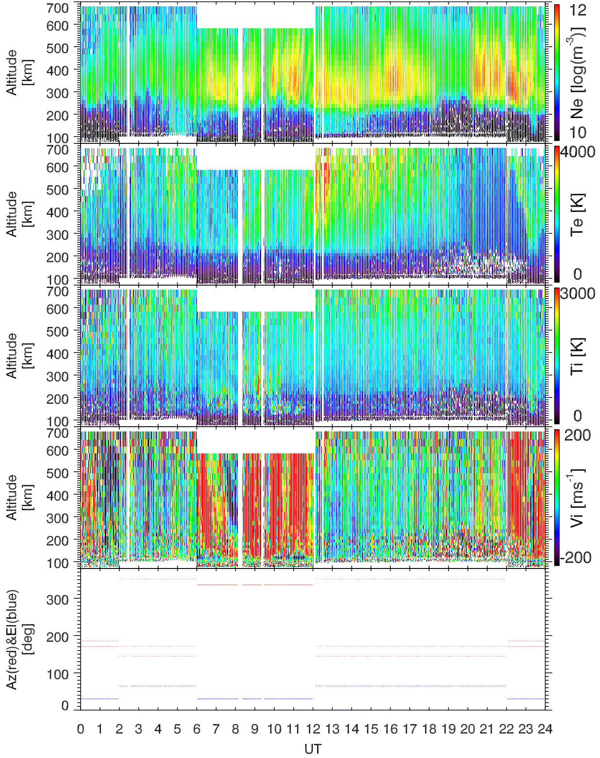
EISCAT 2001-02-20_00_24UT_tau0_ant@32m.
